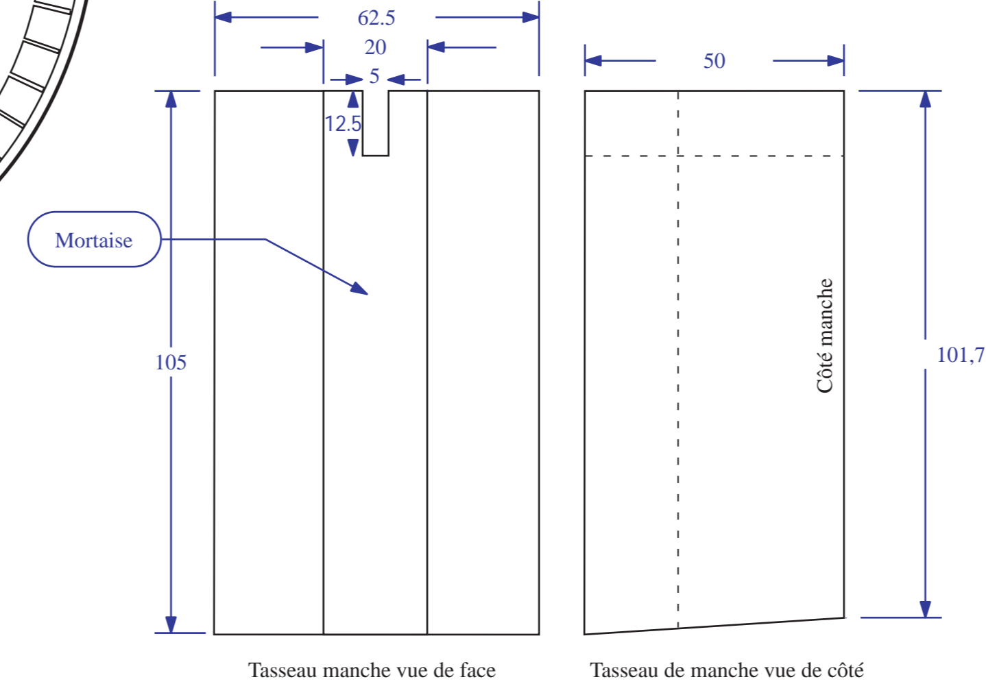
Détail de l'assemblage manche-tasseau de tête
